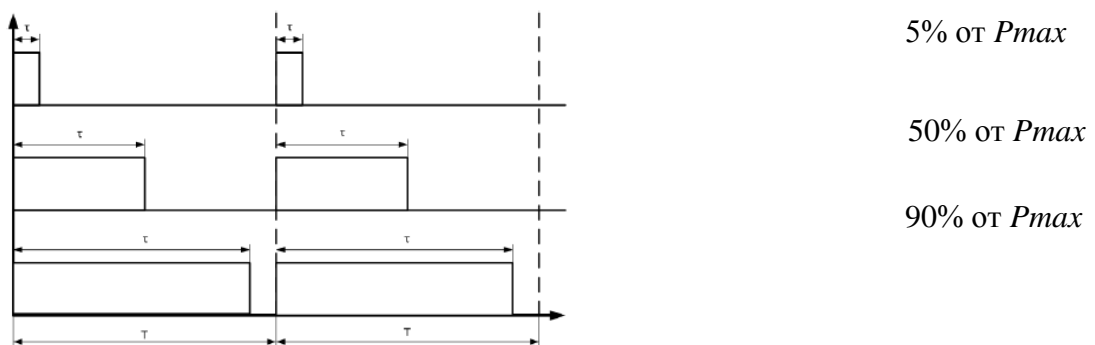
Рис. 3. Принцип действия широтно-импульсной модуляции, P_{max} = 600 Вт
